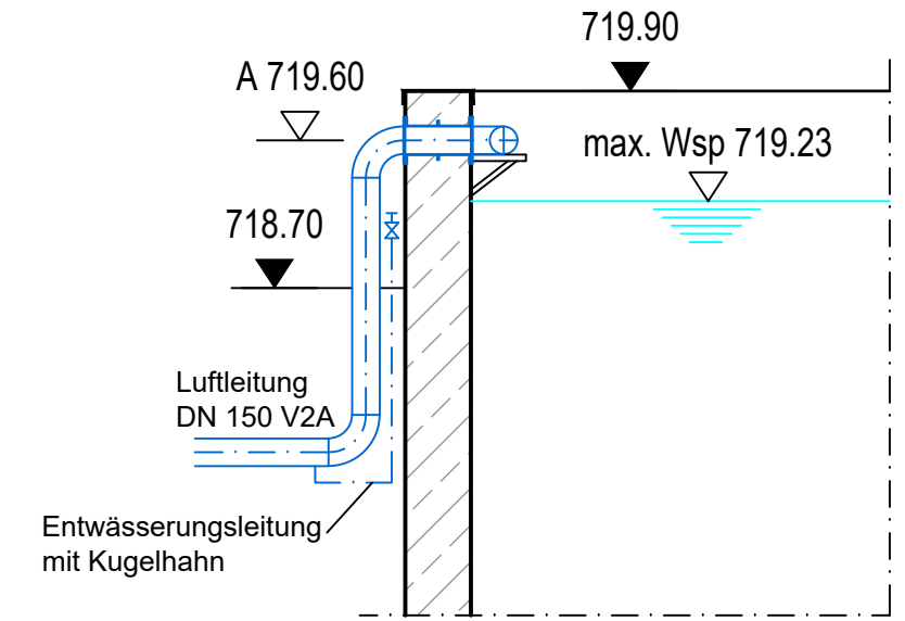
Detail Luftleitung M 1:50
